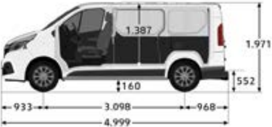
Kastenwagen Frontantrieb (mm) L1H1
